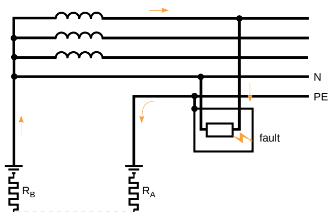
fig. 7: TT-system.
